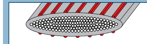
Abb.: Verbesserte Rippenverstärkung
